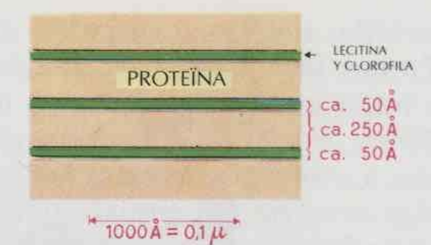
Fig. 3.- Alternancia y dimensiones de los estratos proteínicos y clorofílicos en los grana.
