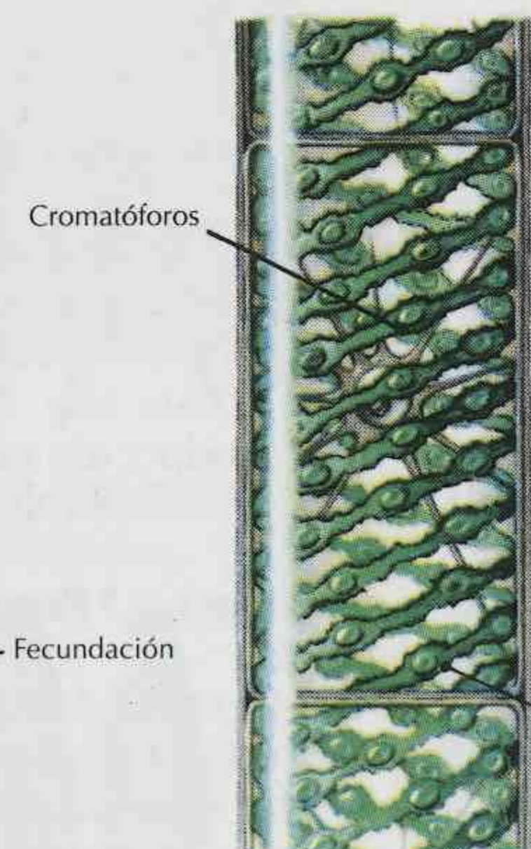
Fig. 7.- Spirogyra crassa .
