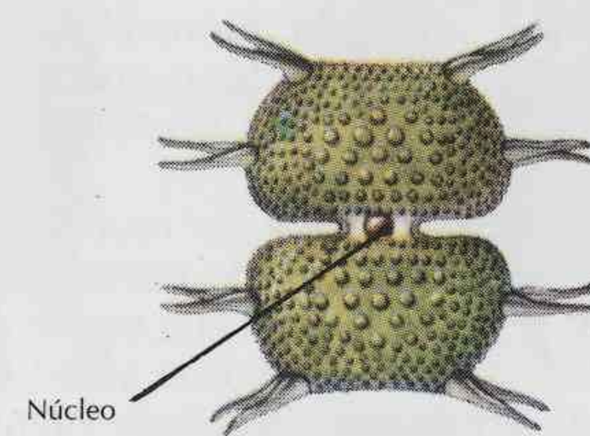
Fig. 4.- Xanthidium fasciculatum .
