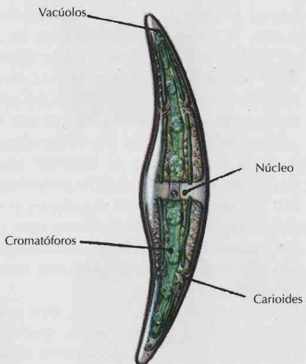
Fig. 5.- Closterium moniliferum .
