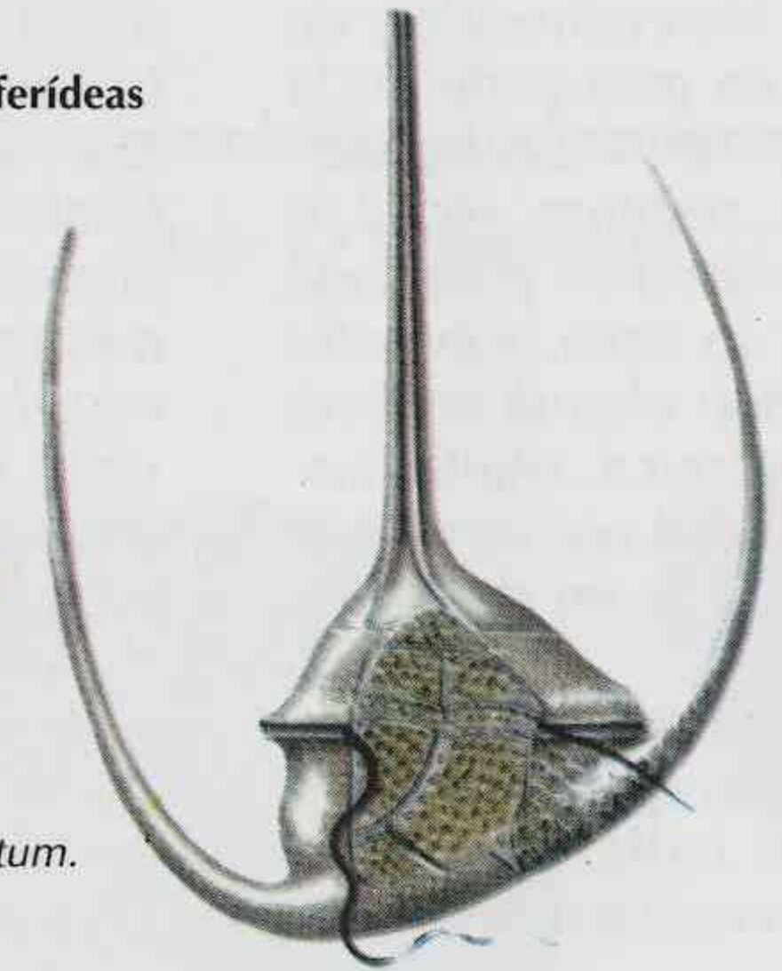
Fig. 8.- Ceratium tripos .
