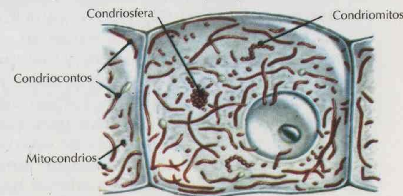
Fig. 8.- Condriosomas.
