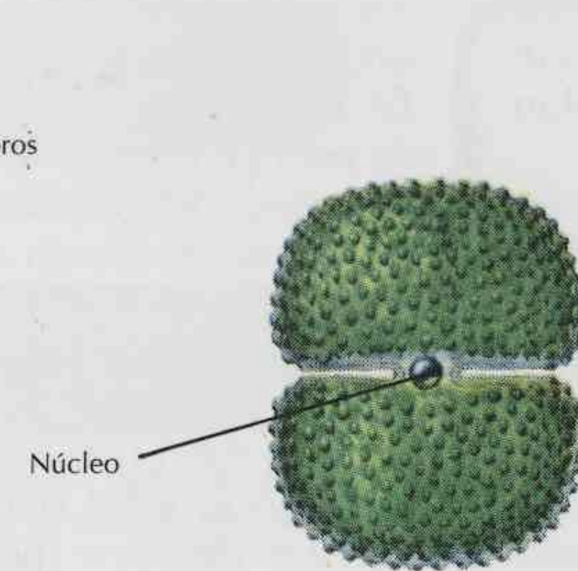
Fig. 2.- Cosmarium sp.
