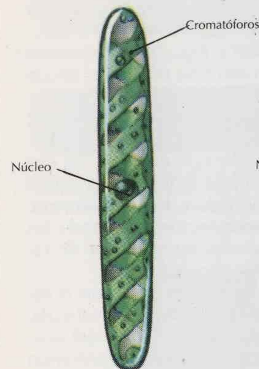
Fig. 1.- Spirotaenia sp.
